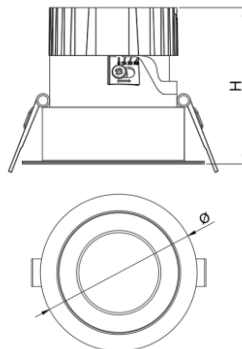
ГАБАРИТНЫЙ ЧЕРТЕЖ
